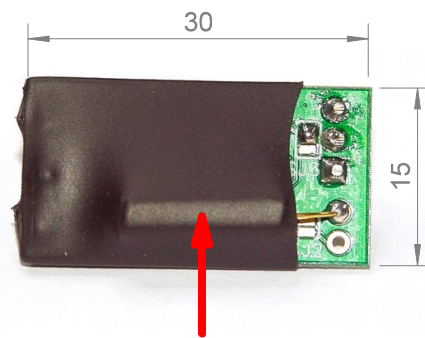
Position Magnetschalter
